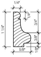
9 STOP DETAIL SCALE: 6" = 1'-0"
