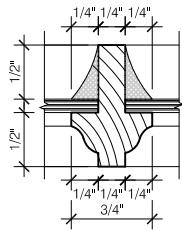
8 MUNTIN DETAIL SCALE: 6" = 1'-0"
