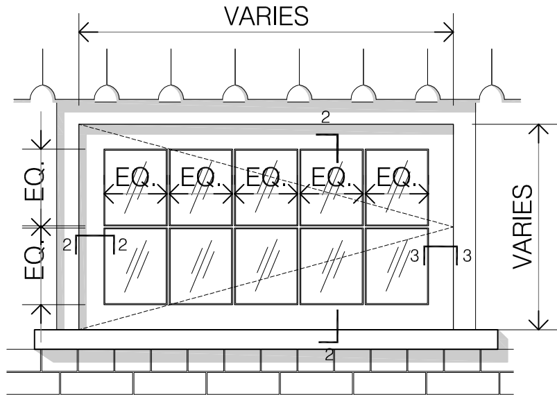
1 WINDOW ELEVATION SCALE: 1" = 1'-0"
