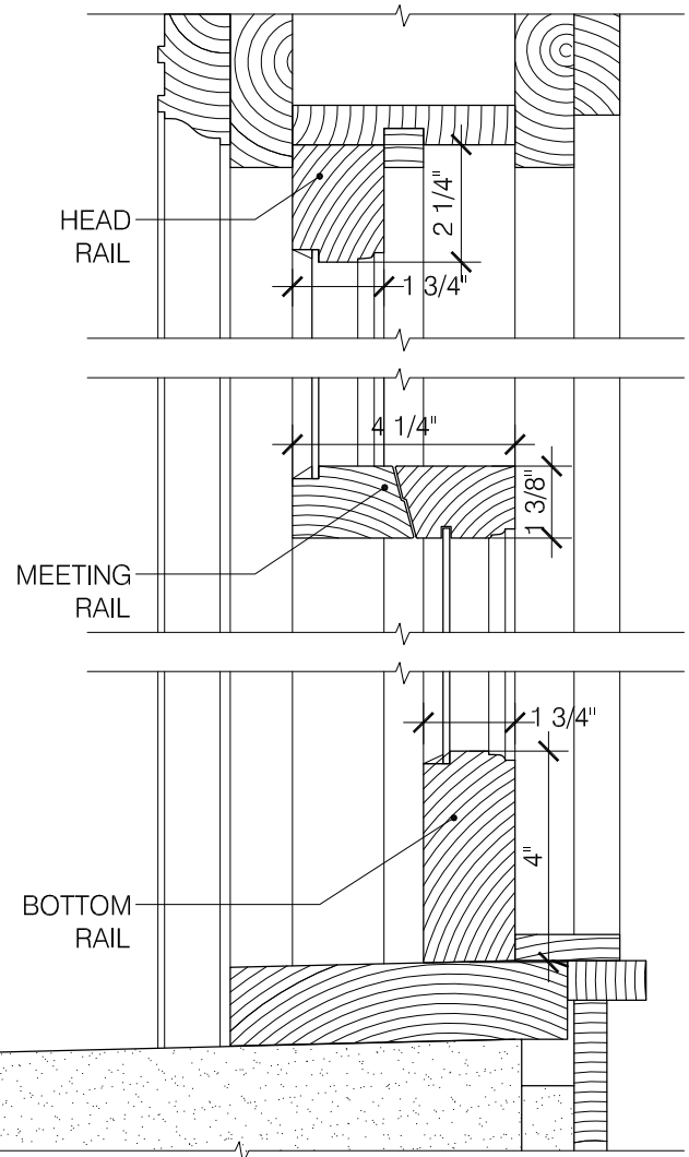
1.1 VERTICAL SECTION SCALE: 3' = 1'-0"
